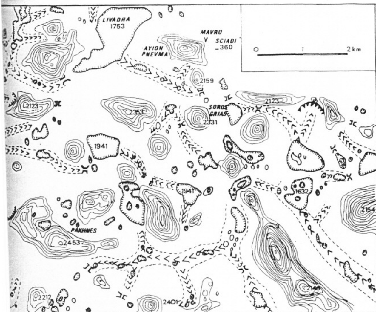
Morphologie du haut karst cônique des Levka Ori (carte du centre du massif).
